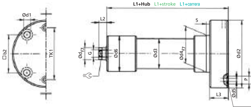
Druckölauführung hinten mit O-Ring-Abdichtung Front of hydraulic fluid connection with o-seal Conexión de fluido hidráulico frontal con junta
