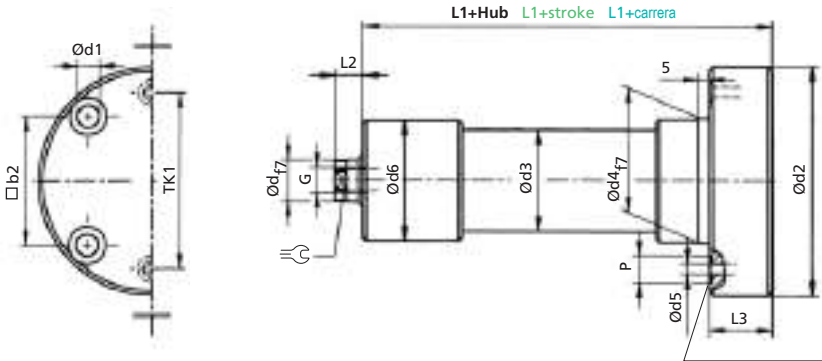
Druckölauführung vorne mit O-Ring-Abdichtung Front of hydraulic fluid connection with o-seal Conexión de fluido hidráulico frontal con junta
