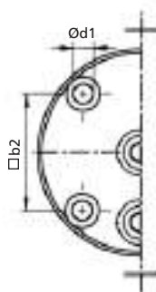
Rohrgewinde-Anschluss hinten Cylinder-thread joint – back view Uniones roscadas del cilindro - vista posterior
