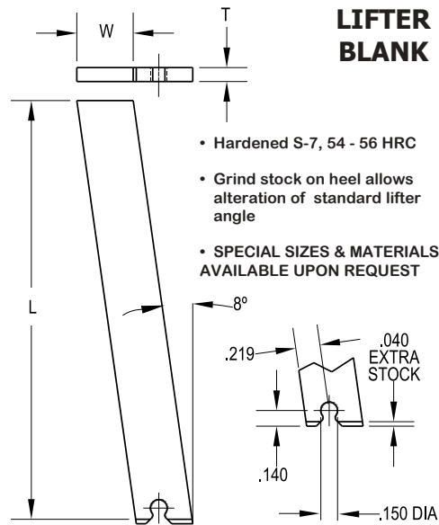
E-Z Lifter™ Mini Lifter Blank Table: Enter custom dimensions below
